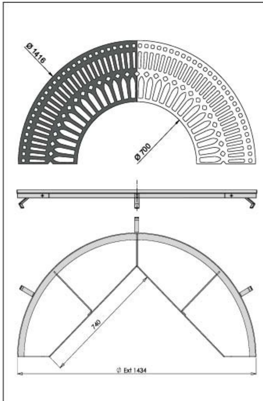
FOURREAU TUTEURAGE
